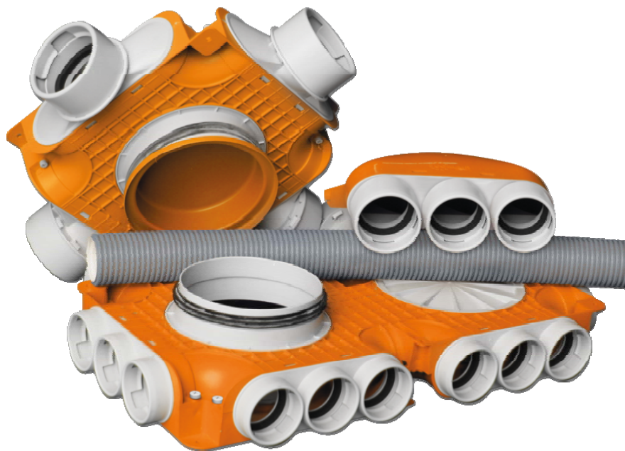
Nowoczesne systemy polietylenowe w 100% można ukryć w przegrodach budowlanych
